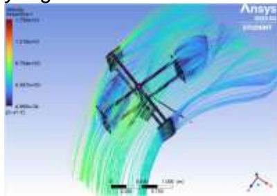
Gambar 4. 13 Velocity Streamline pada turbin 4 bilah kecepatan angin 7 m/s
