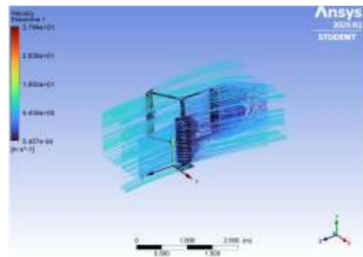
Gambar 4. 11 Velocity Streamline pada turbin 3 bilah kecepatan angin 9 m/s
