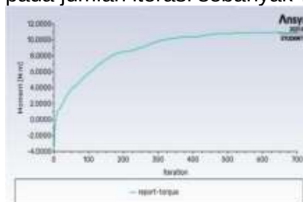
Gambar 4. 6 Grafik torsi turbin 4 bilah pada kecepatan angin 9 m/s
