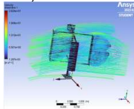
Gambar 4. 15 Velocity Streamline pada turbin 4 bilah kecepatan angin 11 m/s
